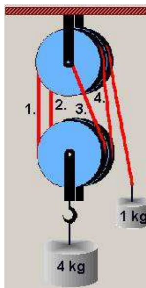
Kladkostroj (obecný)
